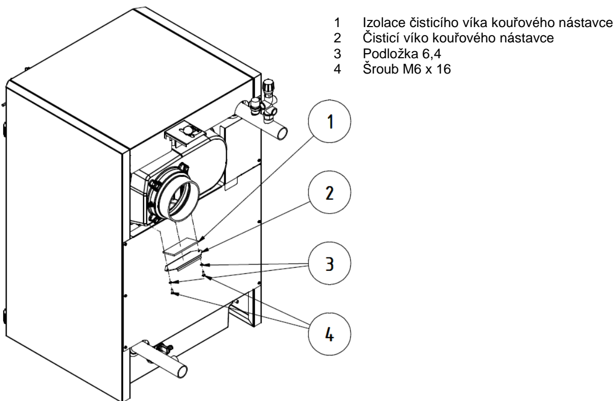
Obr. č. 21 Čištění kouřového nástavce
