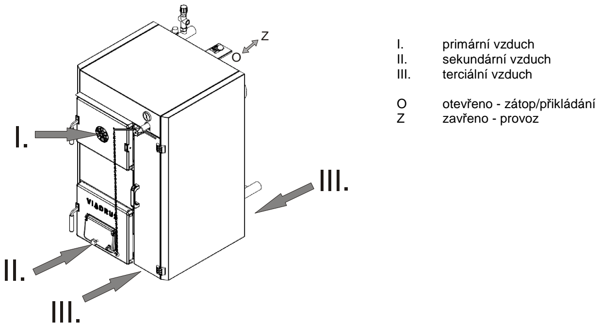
Obr. č. 18 Přívod vzduchů do kotle
