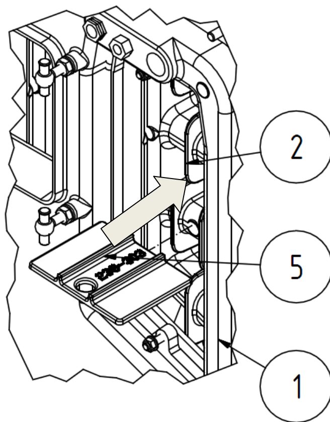
Obr. č. 4 Umístění přepážek spalovacího prostoru
