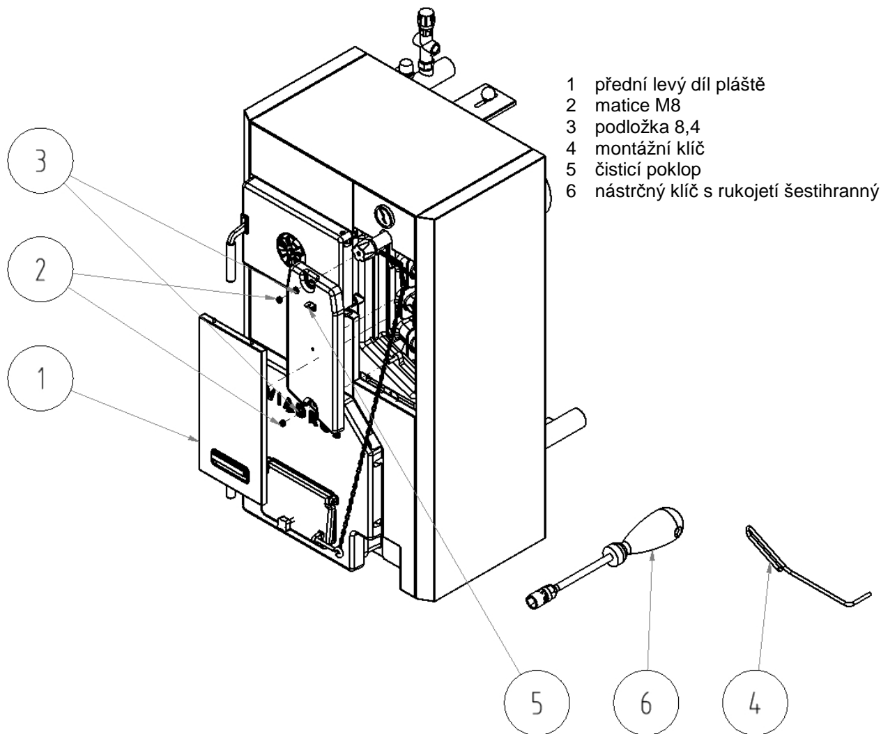
Obr. č. 16 Demontáž čistícího poklopu
