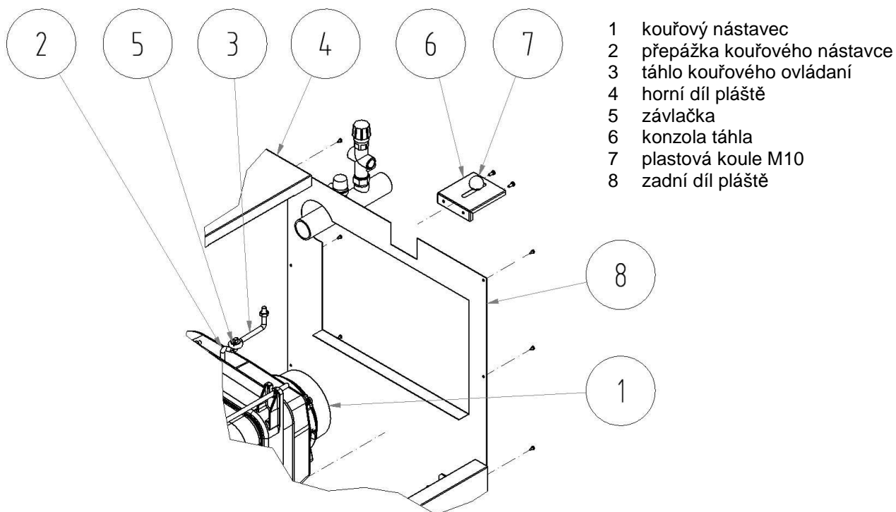
Obr. č. 9 Montáž táhla kouřového ovládaní
