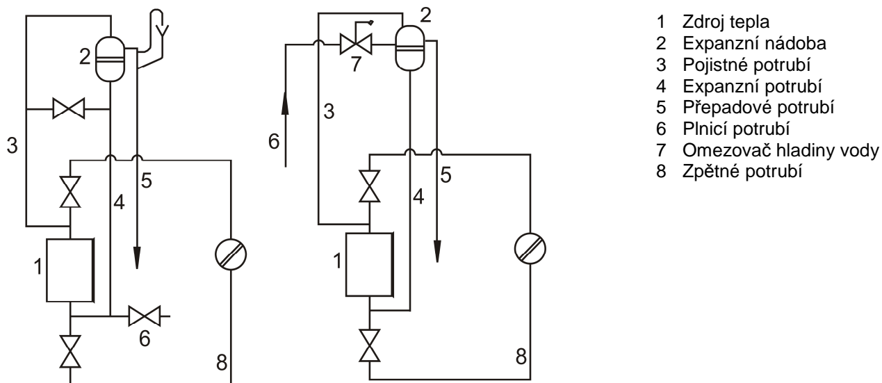
Obr. č. 12 Příklady zapojení otevřených expanzních nádob
