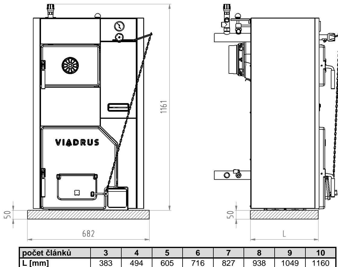
Obr. č. 6 Rozměry podezdívky
