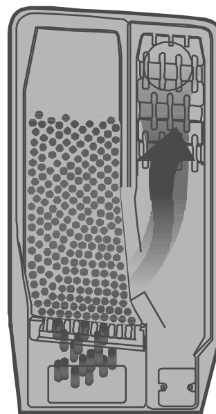
Obr. č. 14 Schéma průchodu spalin kotlem
