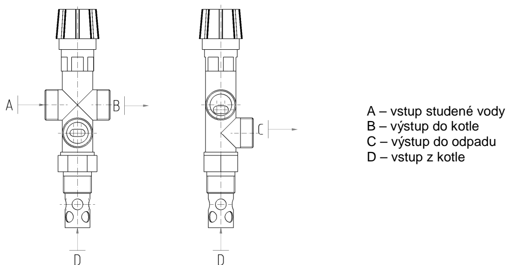
Obr. č. 10 Dvoucestný bezpečnostní ventil DBV 1 – 02
