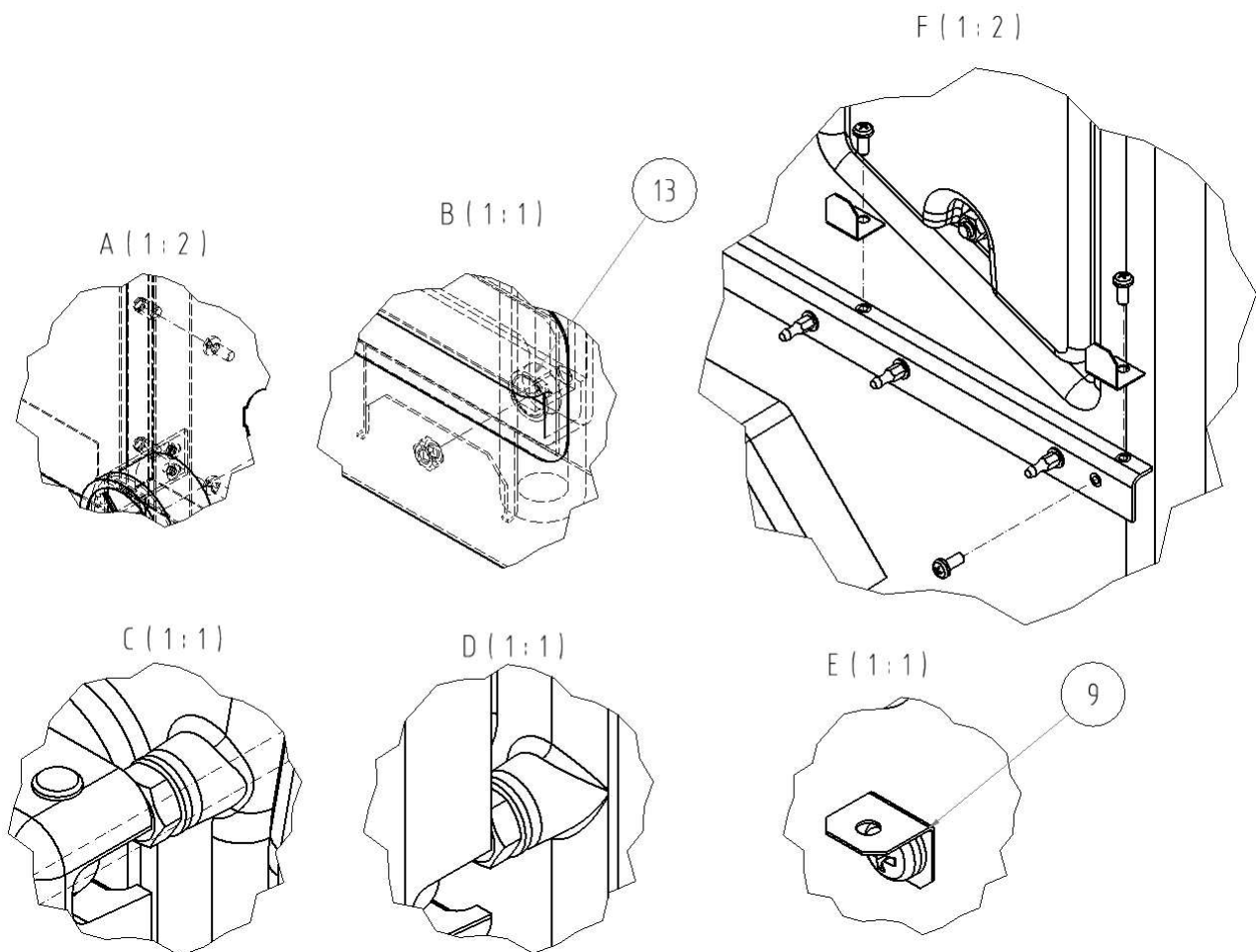
Obr. č. 8 Opláštění kotle
