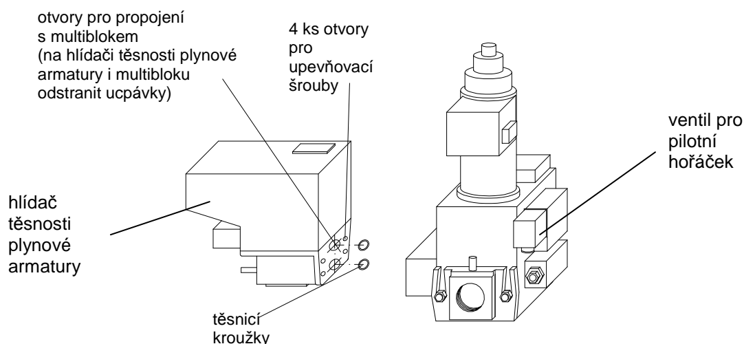
Obr. č. 6 Dvoustupňový elektromagnetický ventil DUNGS MB-ZRDLE 412 s hlídačem těsnosti plynové armatury
