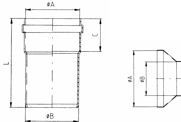
Obr. č. 10 Trubka pro odvod spalin s vyústěním přes zeď \phi 80 a \phi 100 mm mm, tlaková ztráta: 10 Pa
