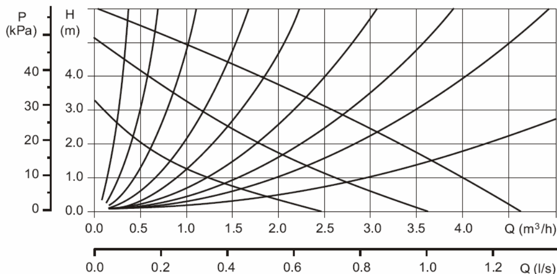
Obr. č. 6 Charakteristika čerpadla UPS 15-60-130
