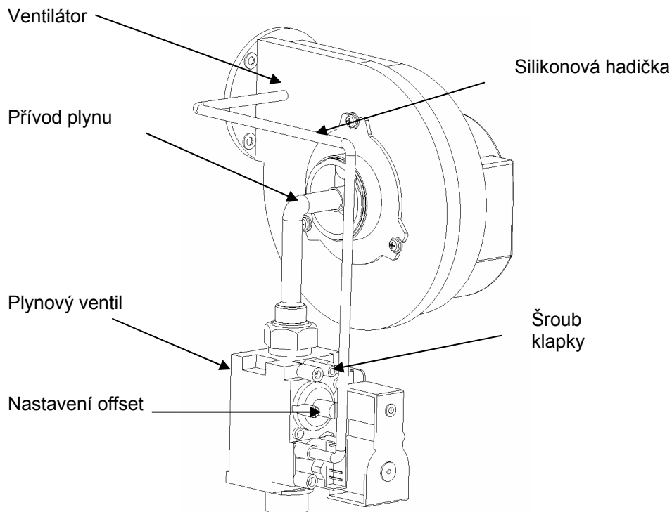
Obr. č. 11 Nastavení K2S pro 2 a 3 čl. velikosti
