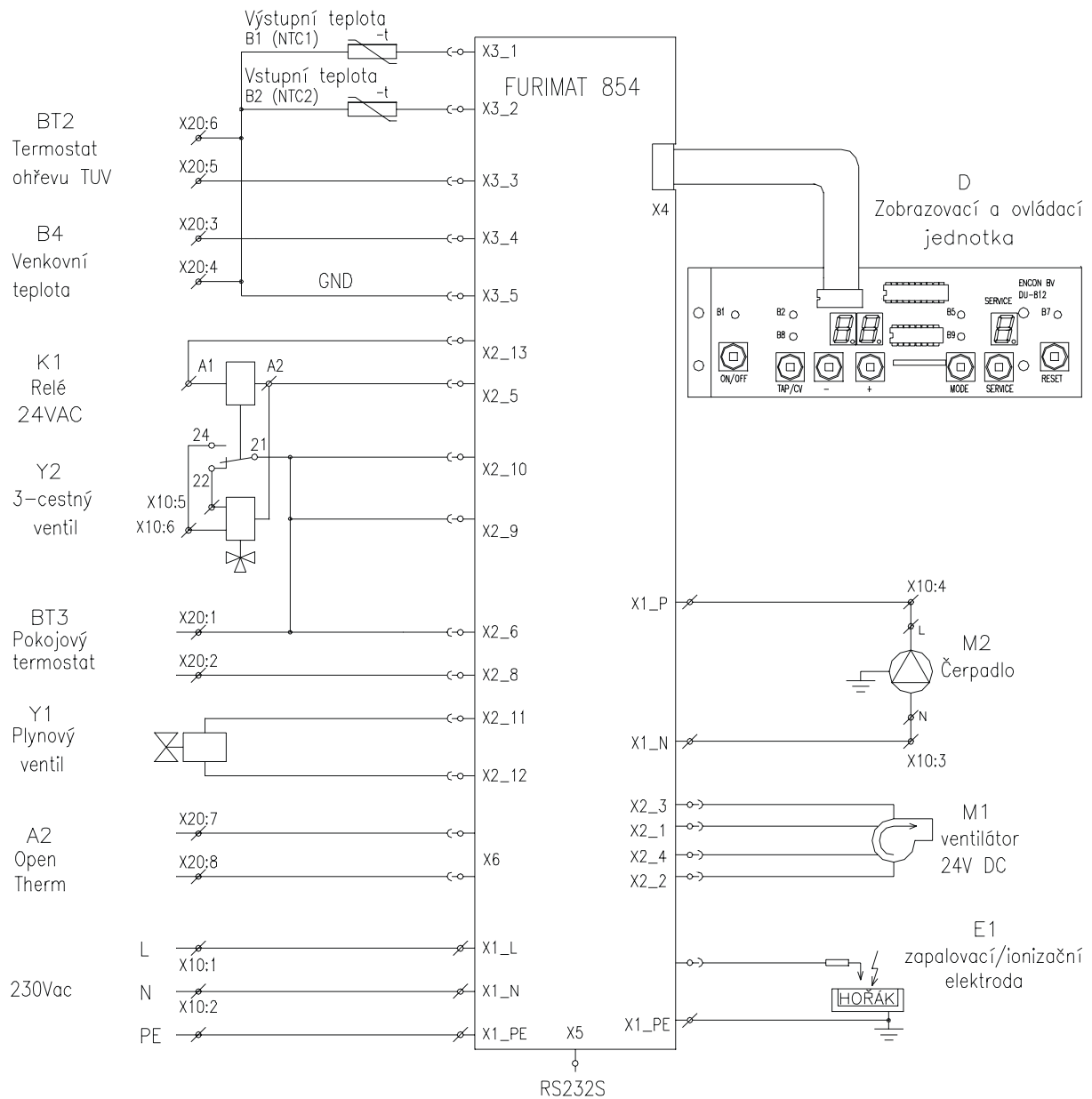
OBVODOVÉ SCHÉMA – CLAUDIUS ( VARIANTA SIT, ČERPADLO+TROJCESTNÝ VENTIL )
