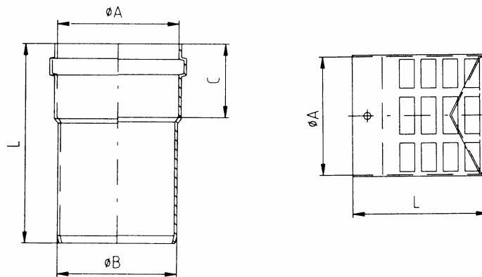
Obr. č. 9 Trubka pro sání vzduchu s vyústěním přes zeď \phi 80 a \phi 100 mm, tlaková ztráta: 15 Pa
