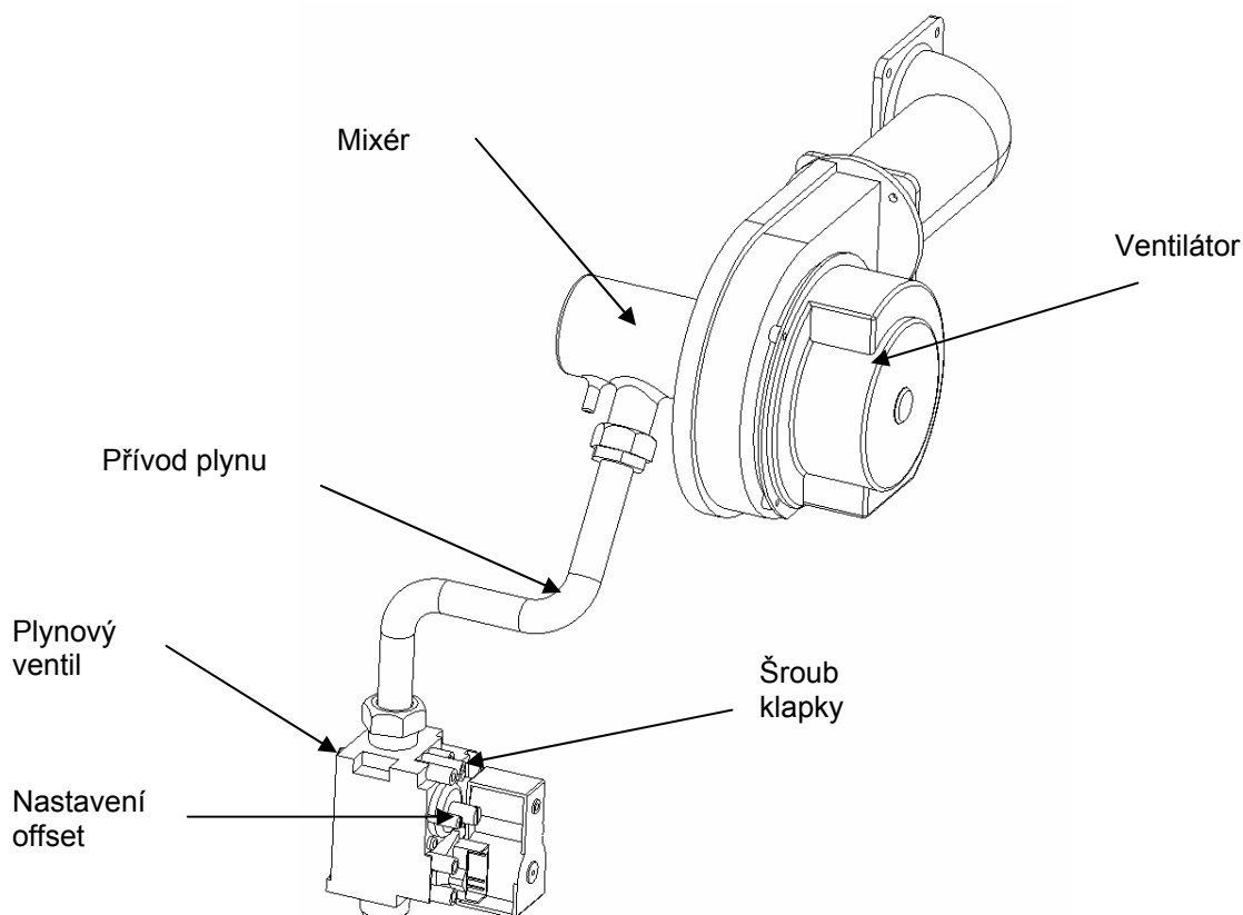
Obr. č. 12 Nastavení K2S pro 5 čl. velikosti
