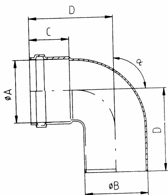
Obr. č. 7 90°koleno \varnothing 80 a \varnothing 100mm, tlaková ztráta 7 Pa
