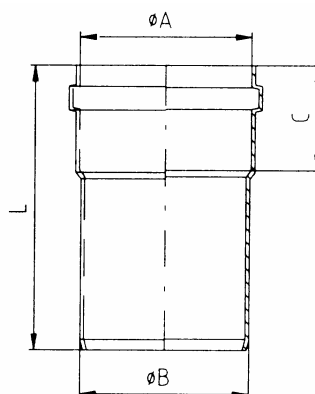
Obr. č. 8 Samostatná prodlužovací trubka vodorovná \varnothing 80 a \varnothing i mm tlaková ztráta: 3,5 Pa
